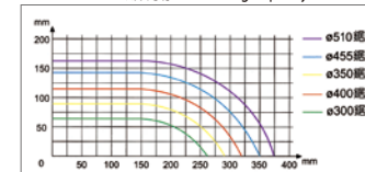
NC-510-3ASE 鋸切能力 Sawing Capacity
