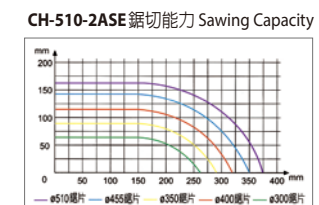
CH-510-2ASE 鋸切能力 Sawing Capacity
